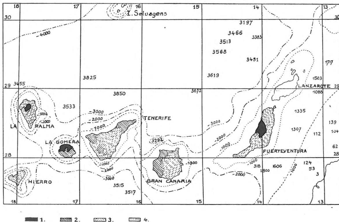
FIG 1. — Groupe des Canaries. — Carte montrant leur position sur le socle continental sous-marin de -3.000 m. et la constitution géologique d'après C. GAGEL.
