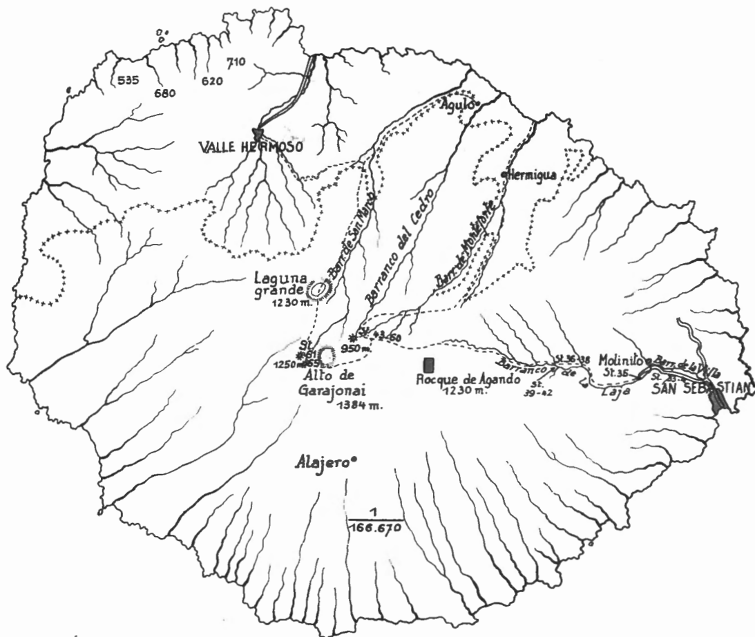
FIG. 16. — La Gomera. — Stations explorées.
